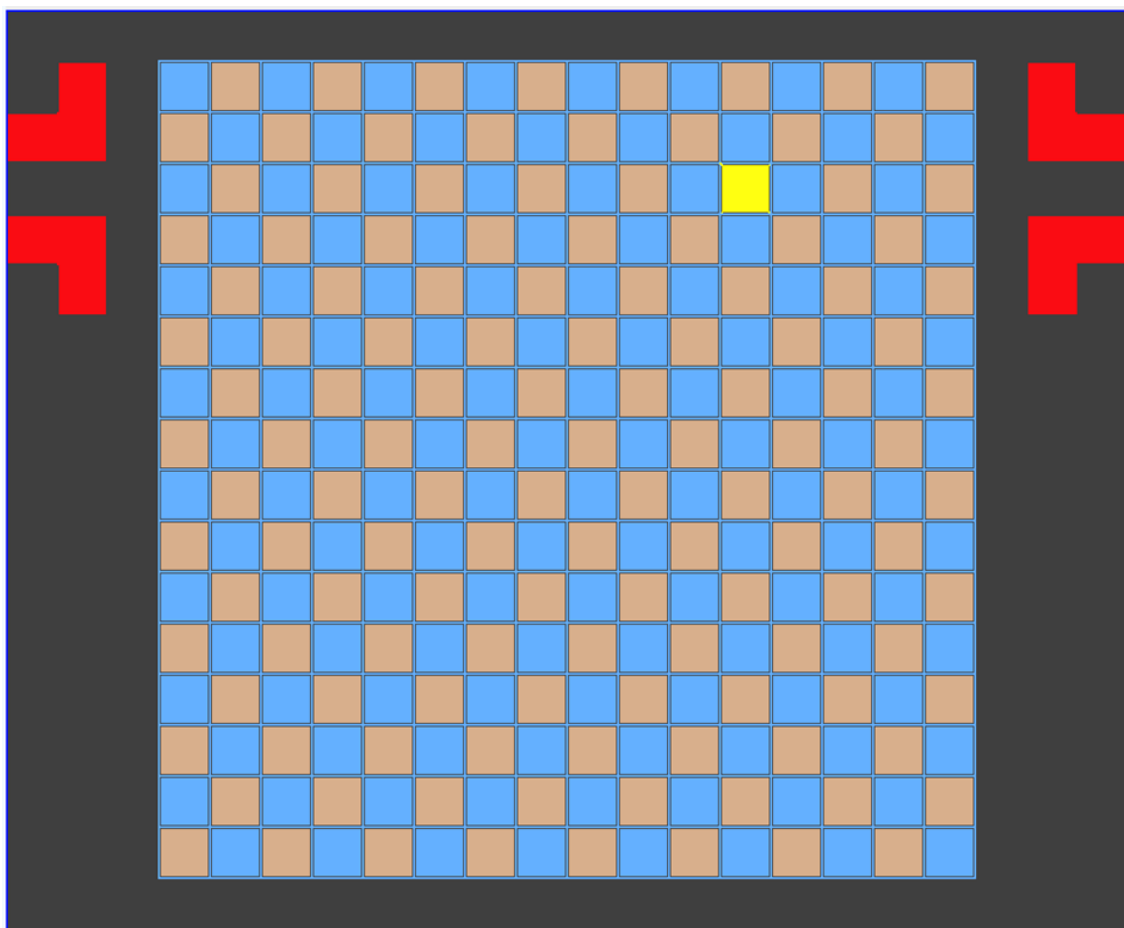
Figure 1: Ein 16 \times 16 -Schachbrett und einige Trominos in rot.
